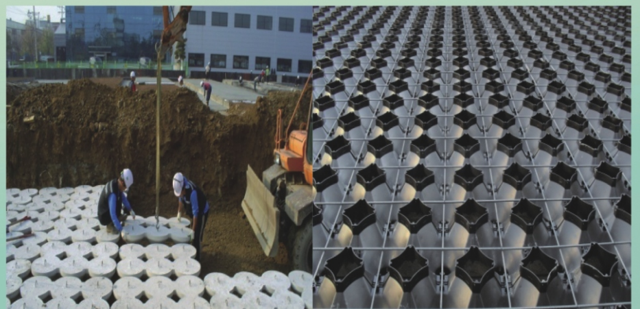
중·저층 건물 지반보강 팡이기초
