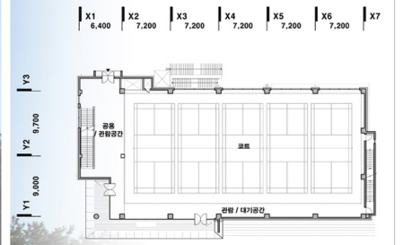
지상 2층 평면도
