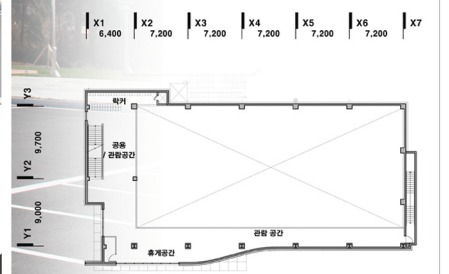
지상 3층 평면도
