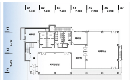
지상 1층 평면도
