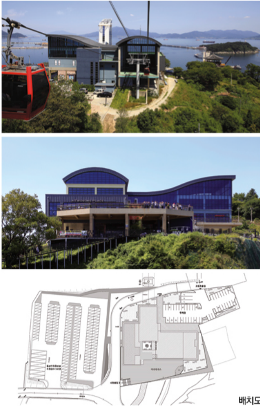
대지위치 : 전라남도 여주시 돌산읍 우두리 산355-134 외 / 대지면적 : 5,722.00㎡ 외 / 건축면적 : 1,790.30㎡ 외 / 연면적 : 4,098.90㎡ 외 용도 : 관광휴게시설 / 규모 : 지하 1층, 지상 3층 / 구조 : 철근콘크리트구조 / 주요 마감 : 에크랄(AL 접합쉬트), 외단열시스템 배치도
