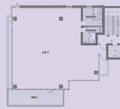
2층 평면도
