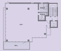
3층 평면도
