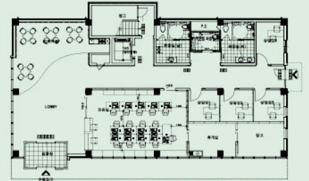
1층 평면도
