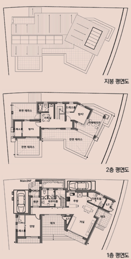
1층 평면도
