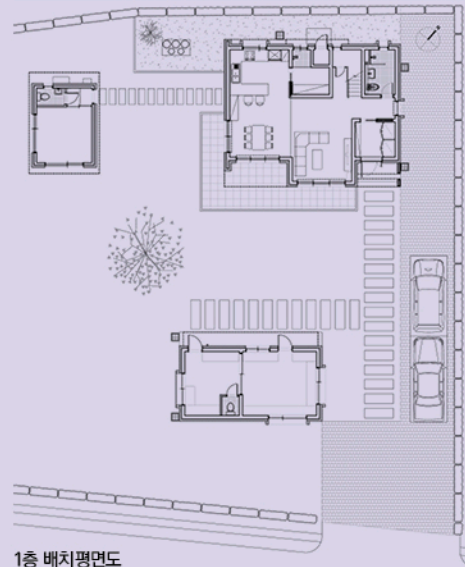
1층 배치평면도
