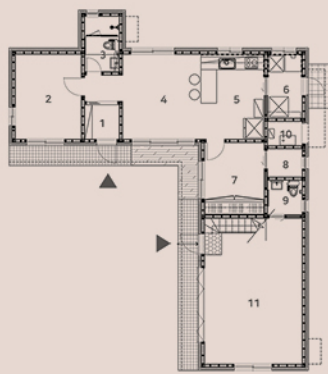
지상 1층 평면도
