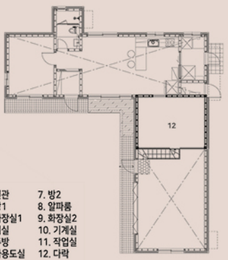
다락층 평면도
