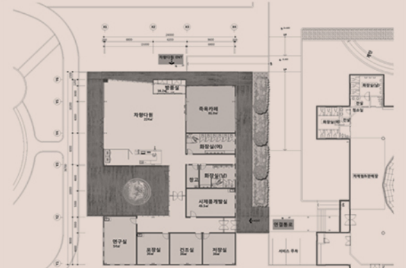
지상 1층 평면도
