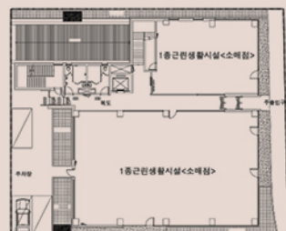
지상 1층 평면도
