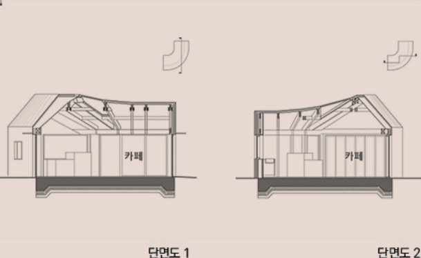
단면도 1
