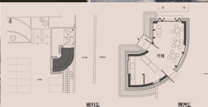
배치도
